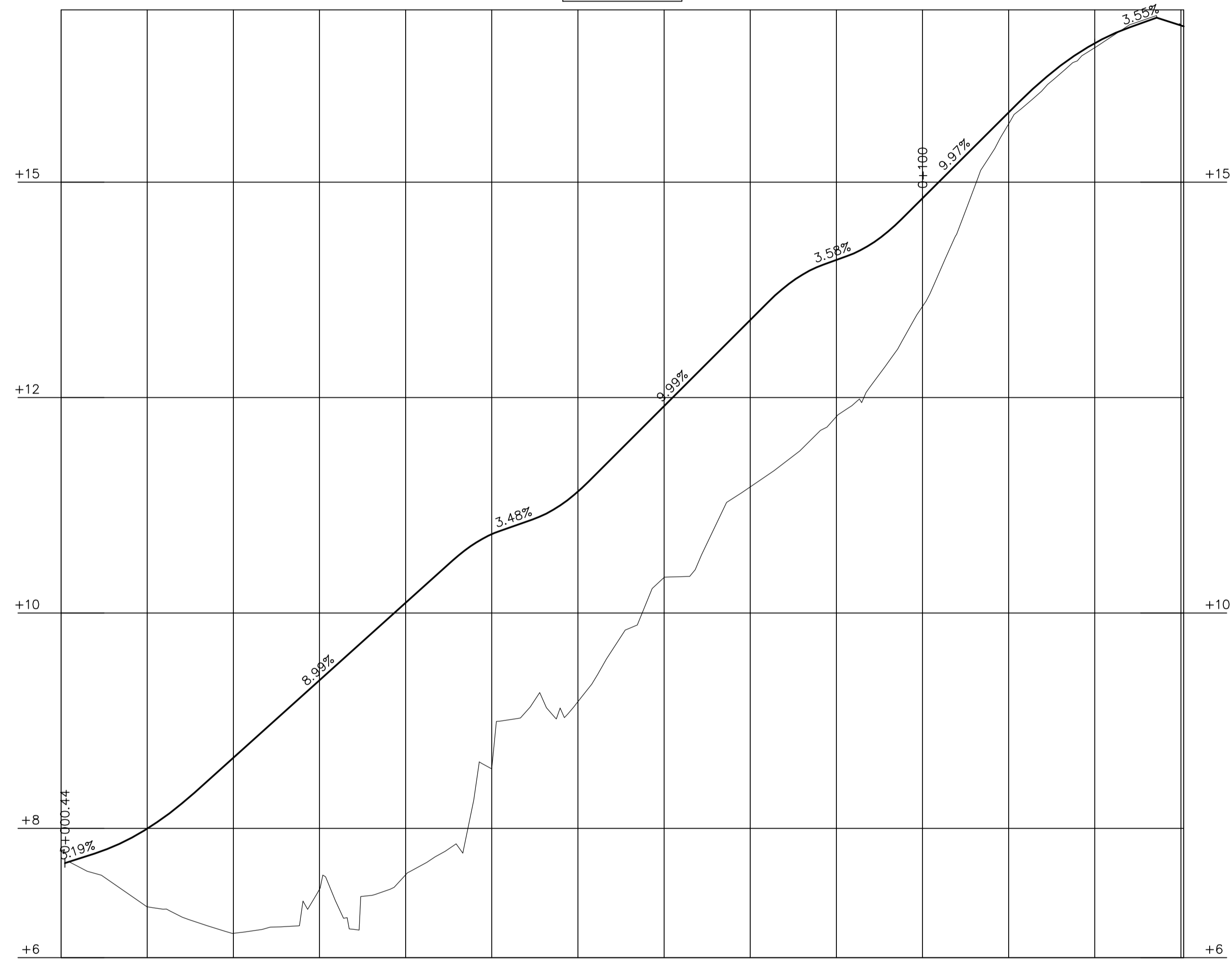
PROFIL: Huvudgata H-SKALA 1:400 V-SKALA 1:40
