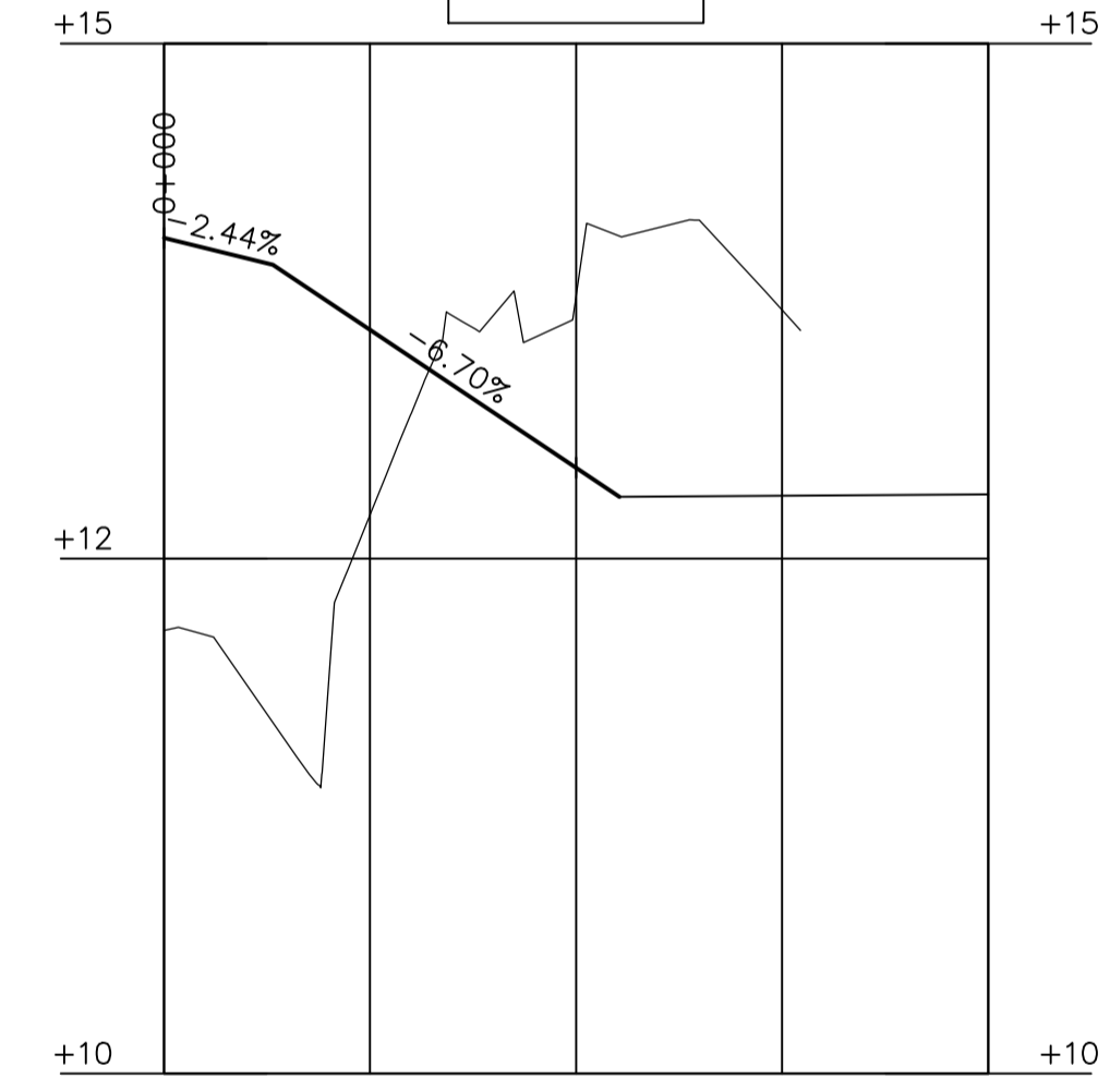
PROFIL: Pilen 19 H-SKALA 1:400 V-SKALA 1:40
