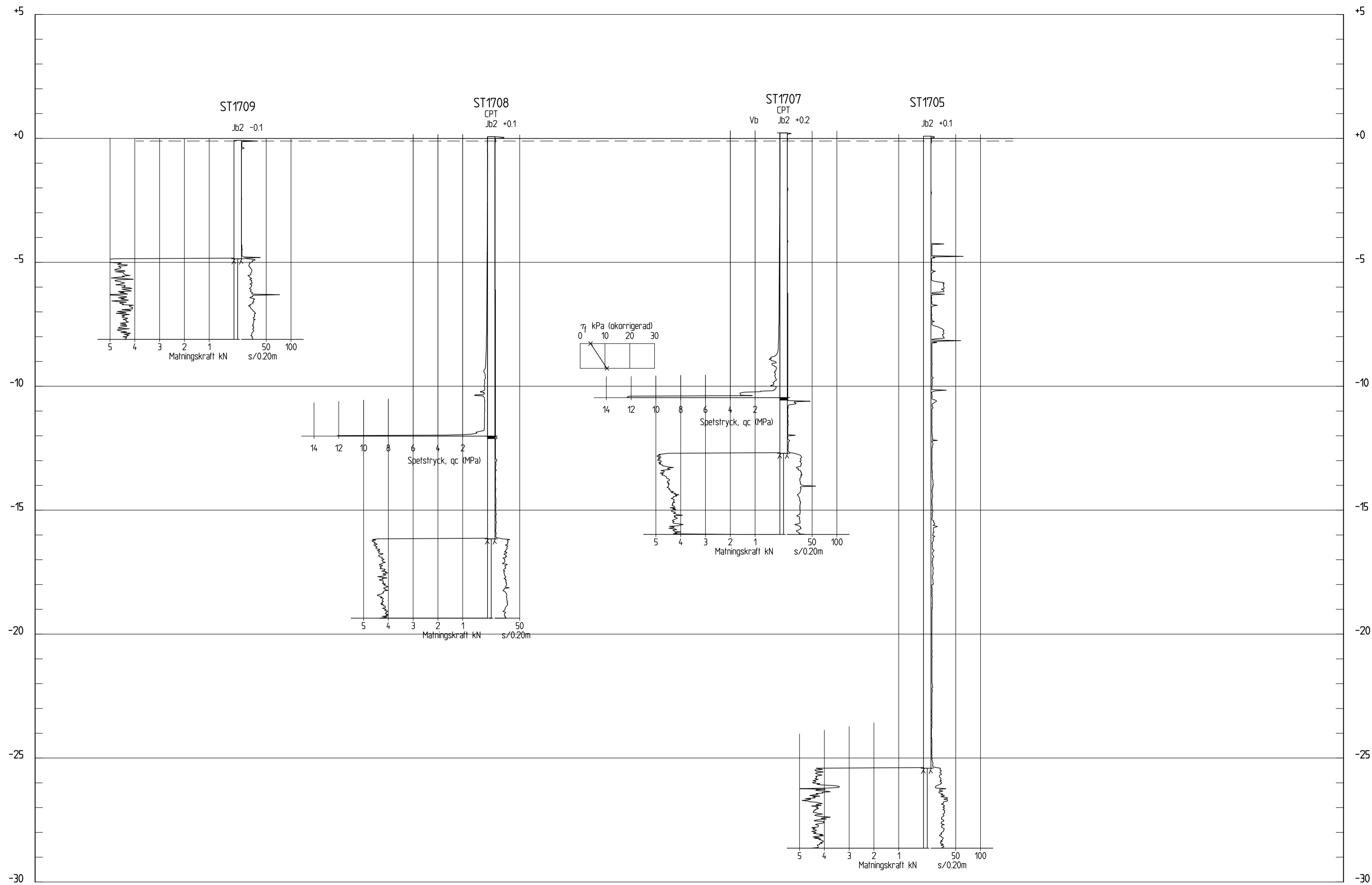
SEKTION J-J H 1: 100 L 1: 200
