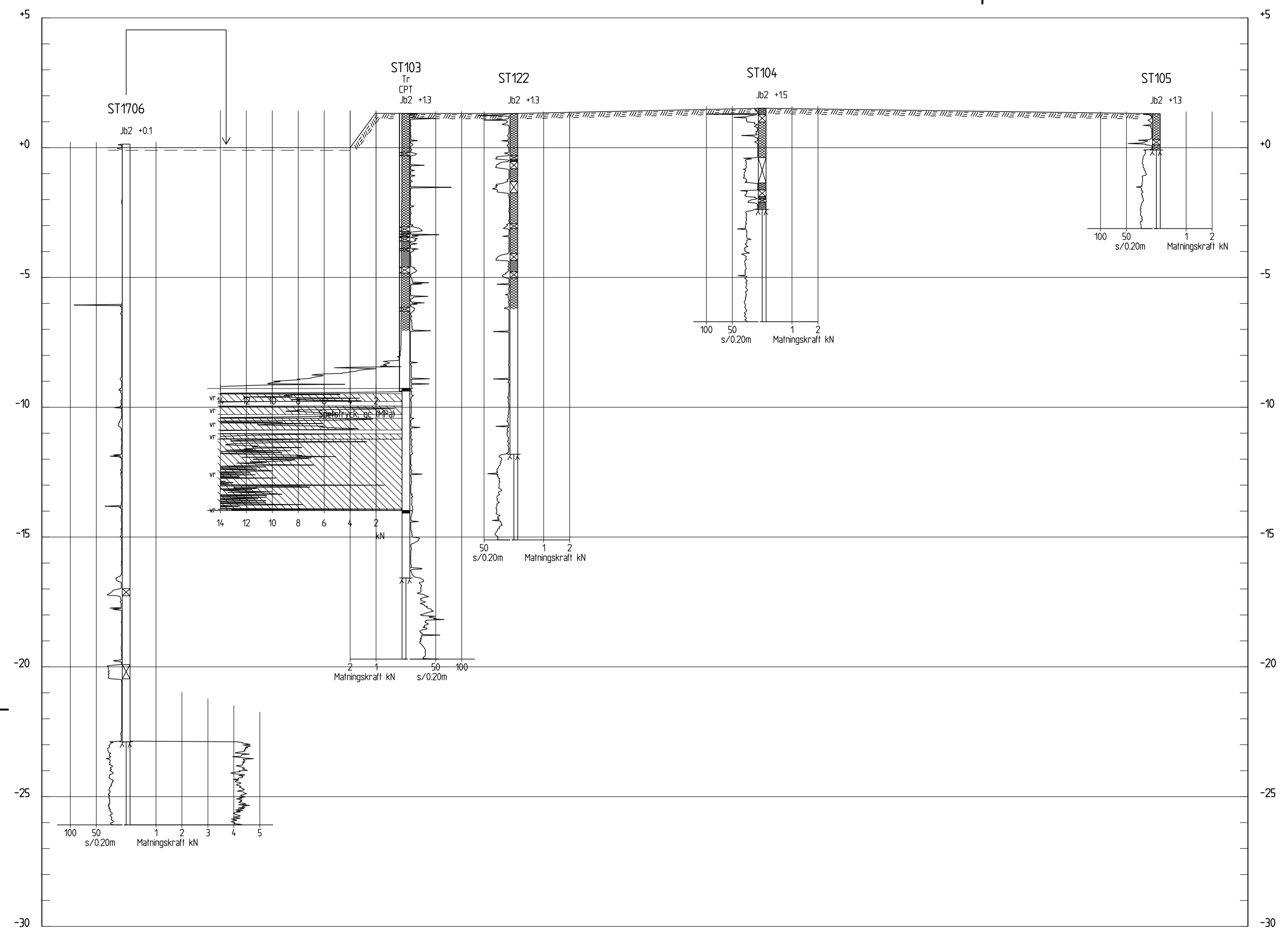
SEKTION A-A H 1: 100 L 1: 200
